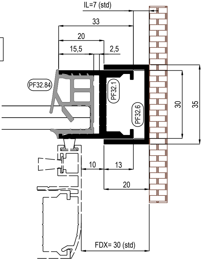
A NODO DI CODA SCALA 1:1 ANTA FISSA
