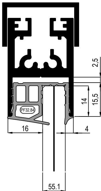
C STRATIFICATO 55.1
