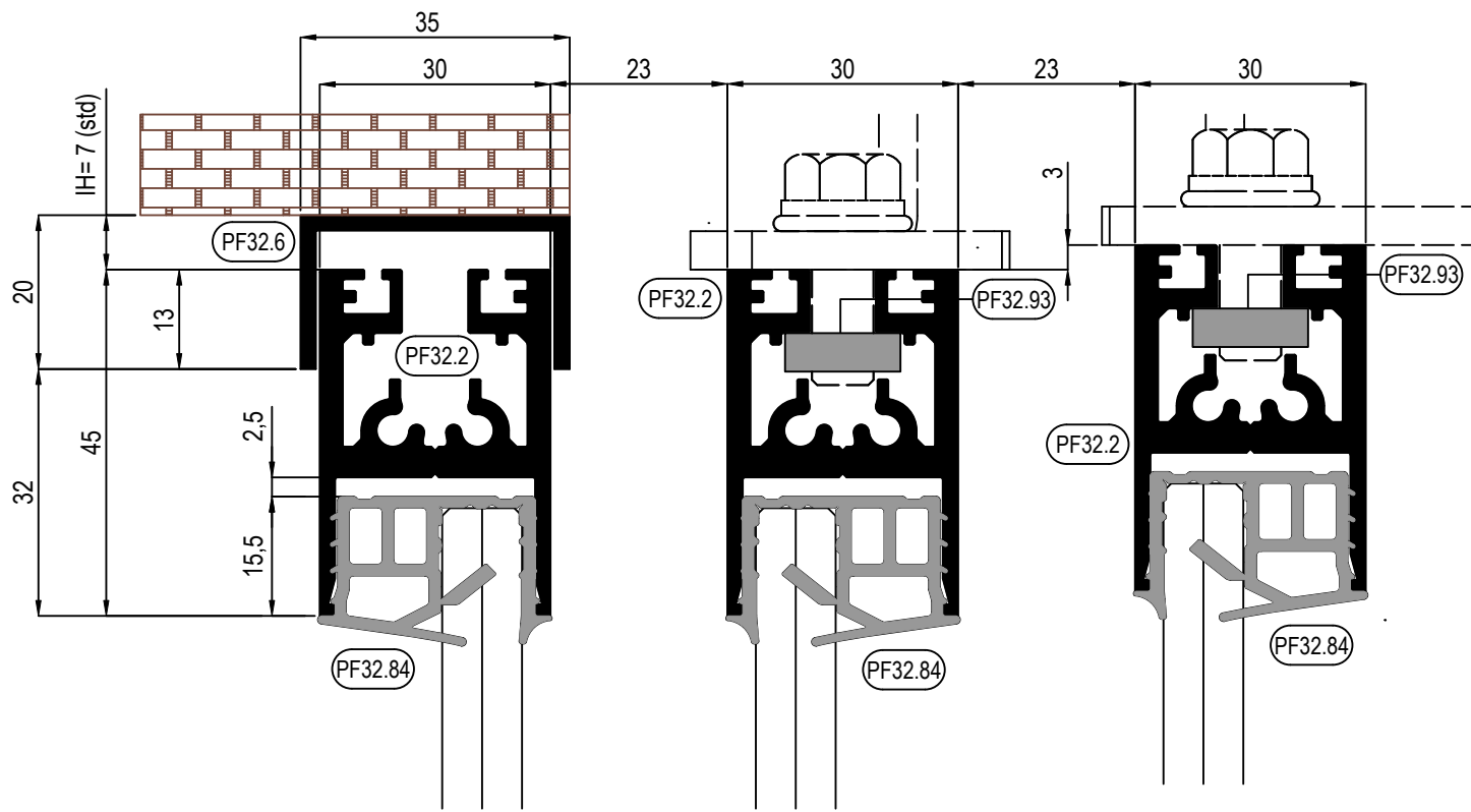
SEZIONE CON VETRO STRATIFICATO PER ULTERIORI VETRI VEDI CAPITOLO VETRAZIONE
