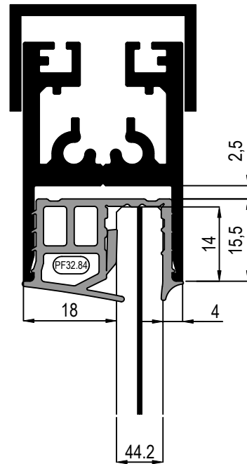
B STRATIFICATO 44.2
