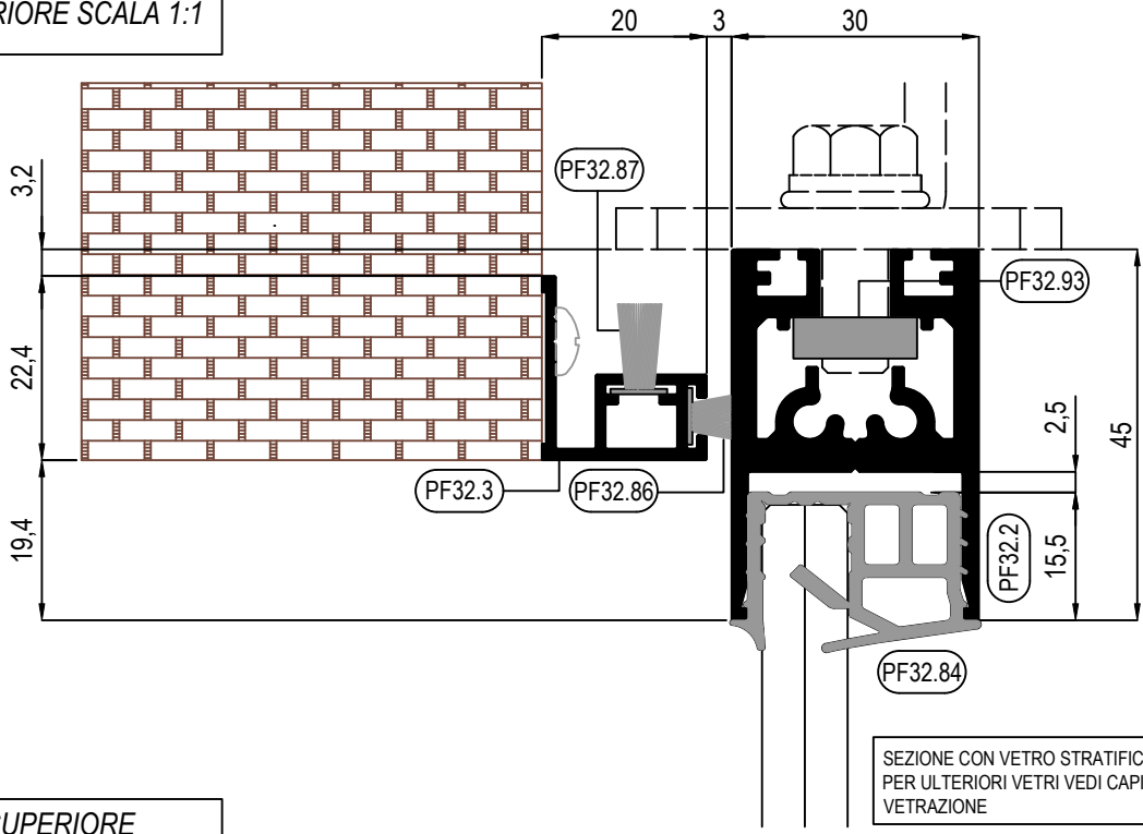
OPZIONE CON GUARNIZIONE DI TENUTA
