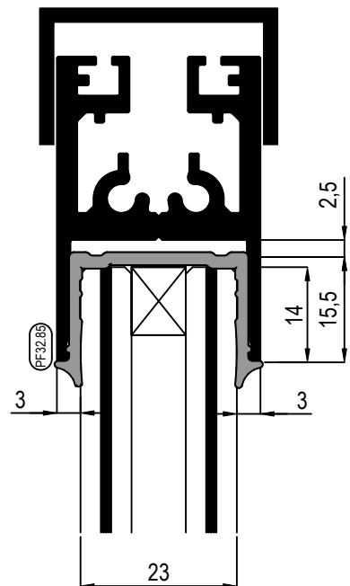
H CAMERA ANTIINTRUSIONE PA4 (EN356) 33.4/8/33.4
